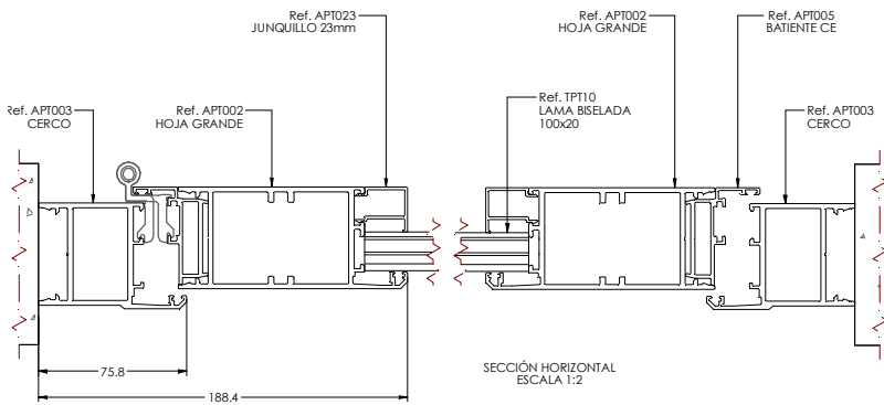
Puerta de paso peatonal abatible de 1 hoja. Sección horizontal.
