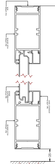
Puerta de paso peatonal abatible. Sección vertical.
