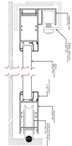
Puerta de paso peatonal corredera, motorizada. Sección vertical.
